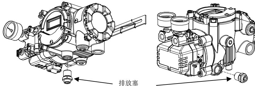
图3-1: 排放塞位置与定位器安装支座方向对应
