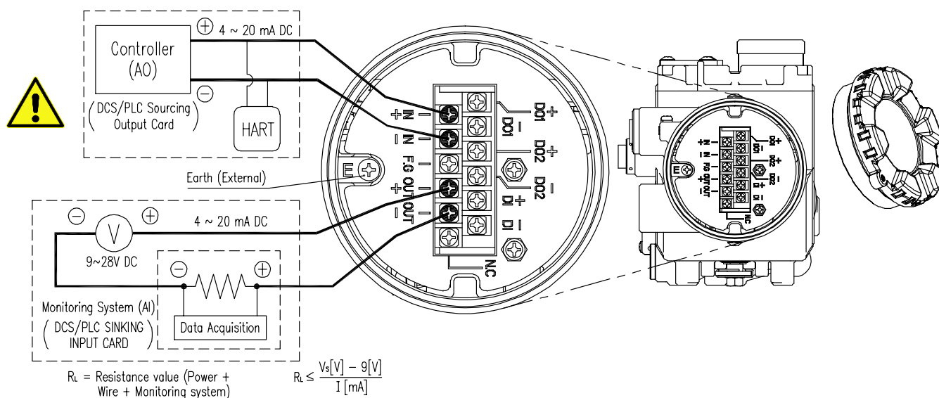
图5-3: 端子概览1
