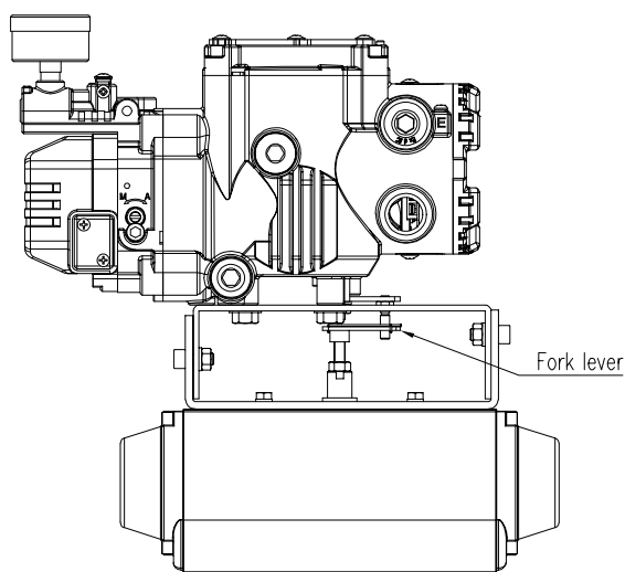
图3-11: 叉杆型
