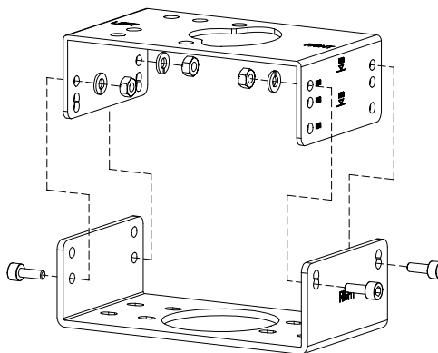
图3-15: 支架分解图
