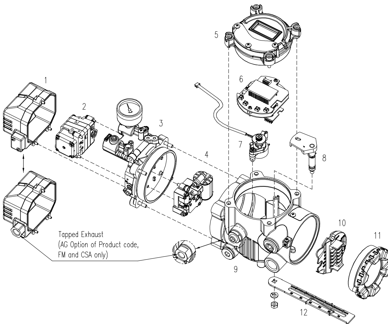
图2-1: 分解图
