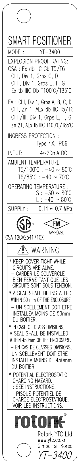
图L-4: YT-3400, 3450金属标签 (适用于FM, CSA)
