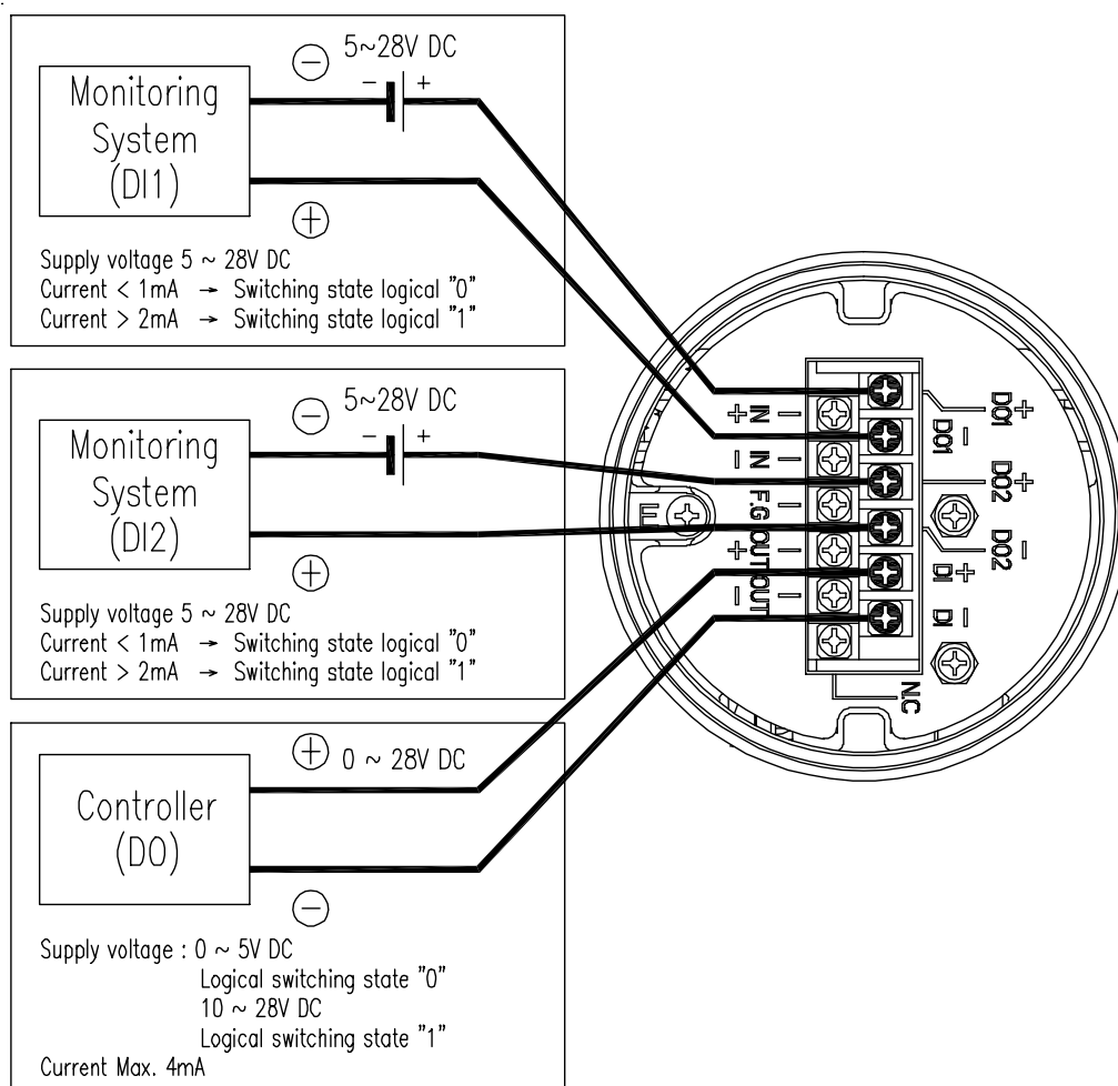
图5-4: 端子概览2
