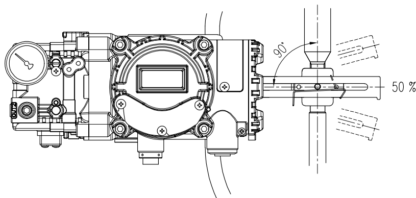
图3-8: 反馈杆和阀杆
